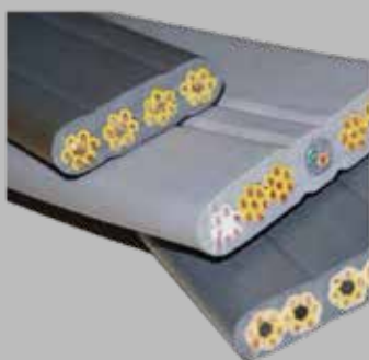
CABLE VIAJERO 12-24-40 HILOS
